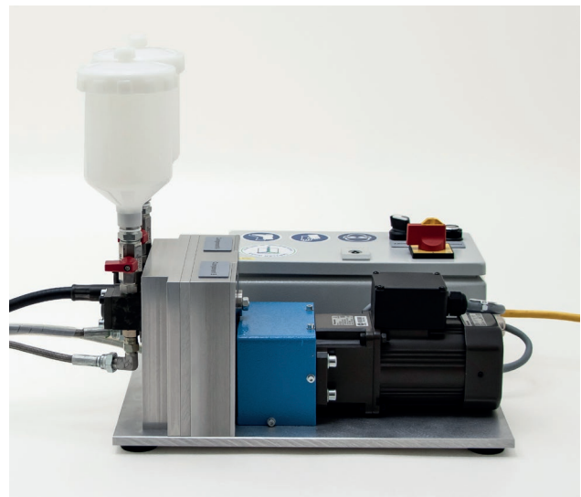
Ausführungsbeispiel einer MDM 4 mit 0,6 l Behältern.
